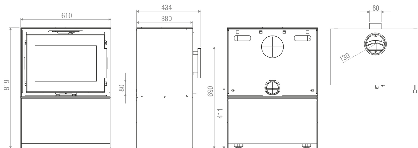
Schéma technique
