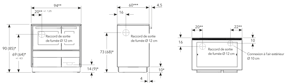
Appareil sur pied avec étuve
