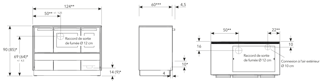
Appareil sur pied avec étuve
