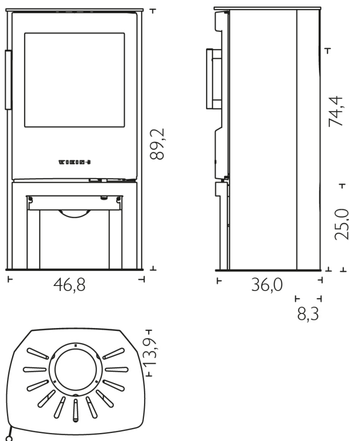
Schéma technique
