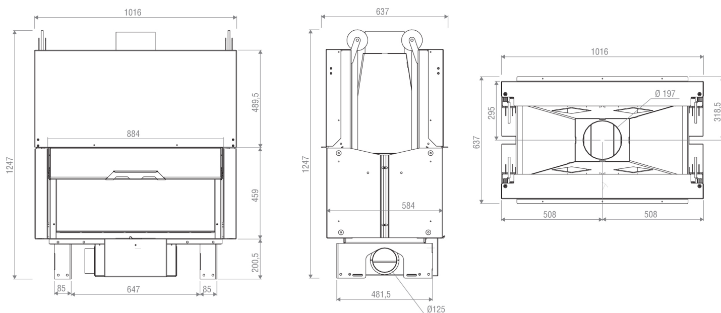
Schéma technique
