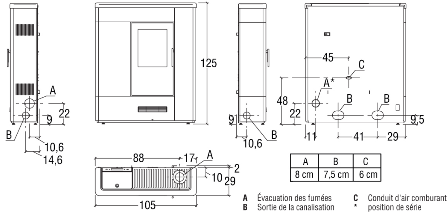
Schéma technique
