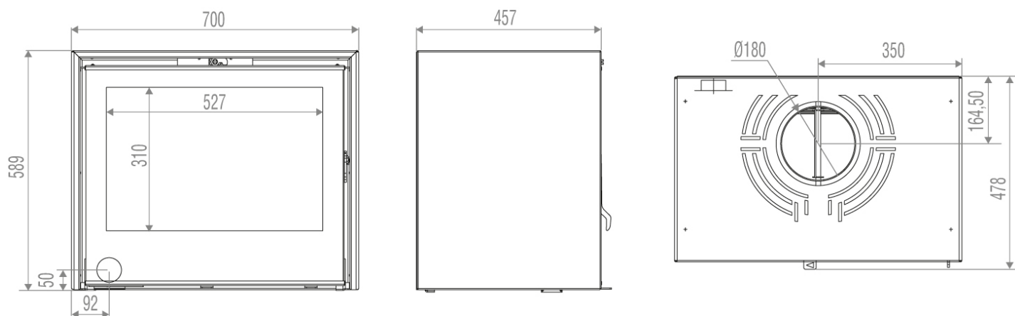
Schéma technique
