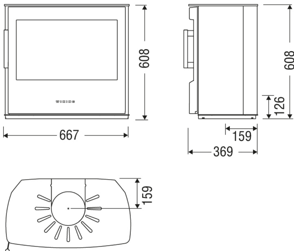
Schéma technique
