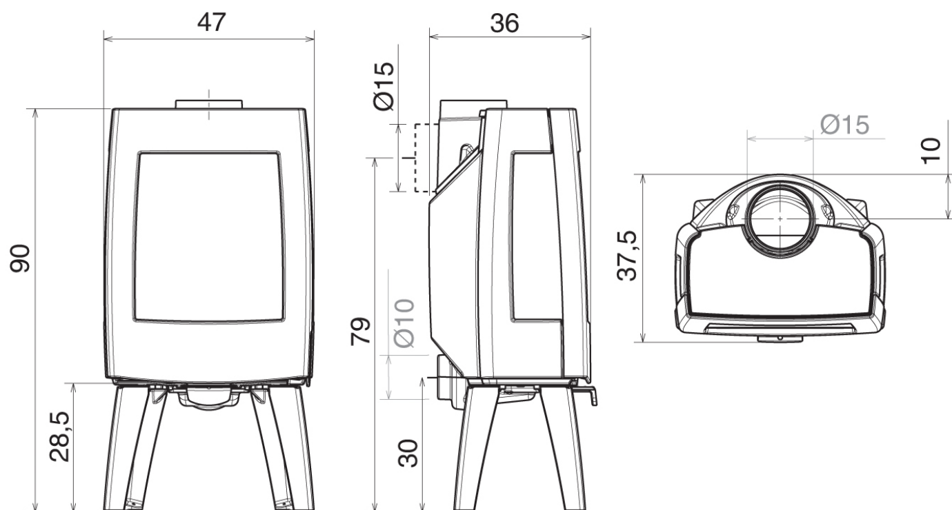
Schéma technique
