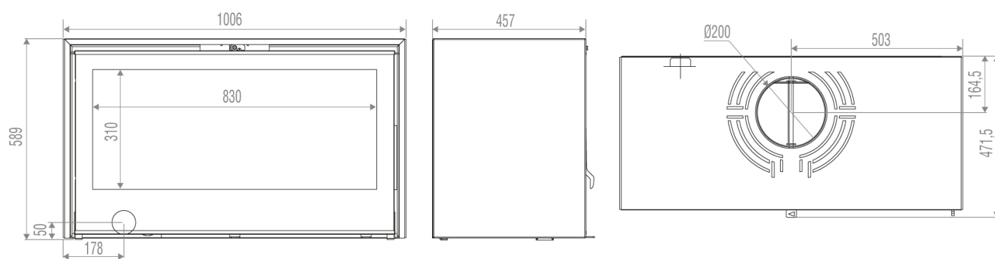
Schéma technique
