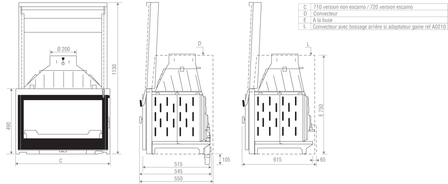
Schéma technique
