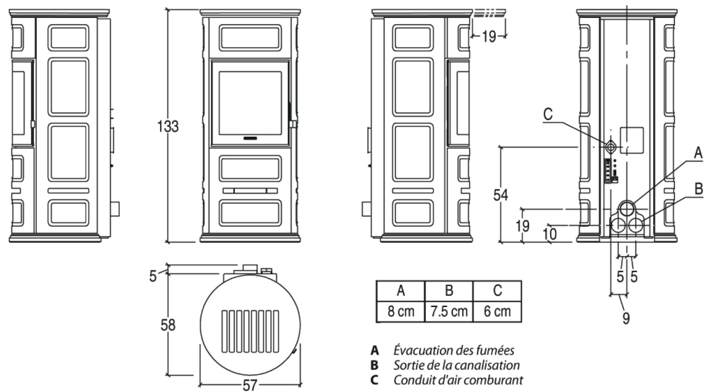
Schéma technique
