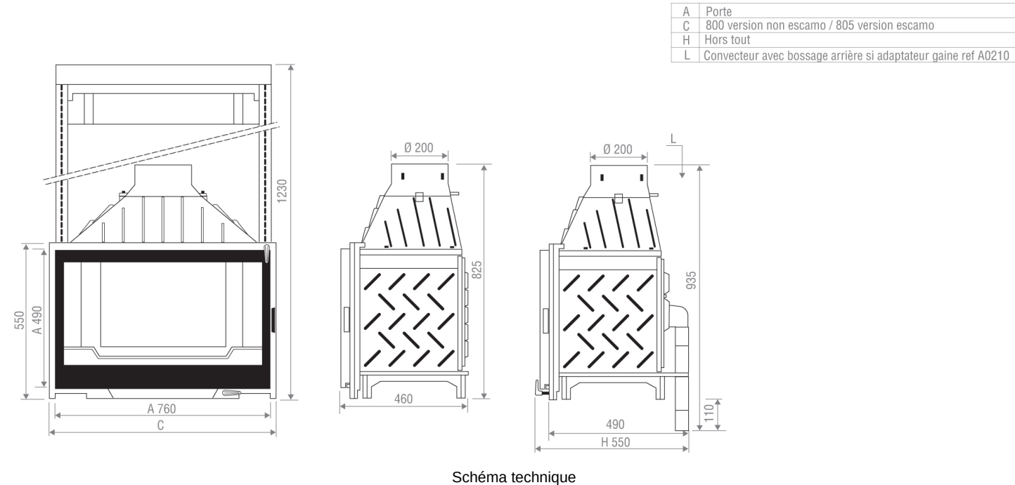
Schéma technique
