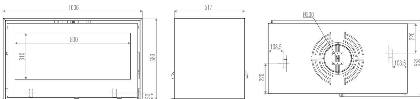
Schéma technique
