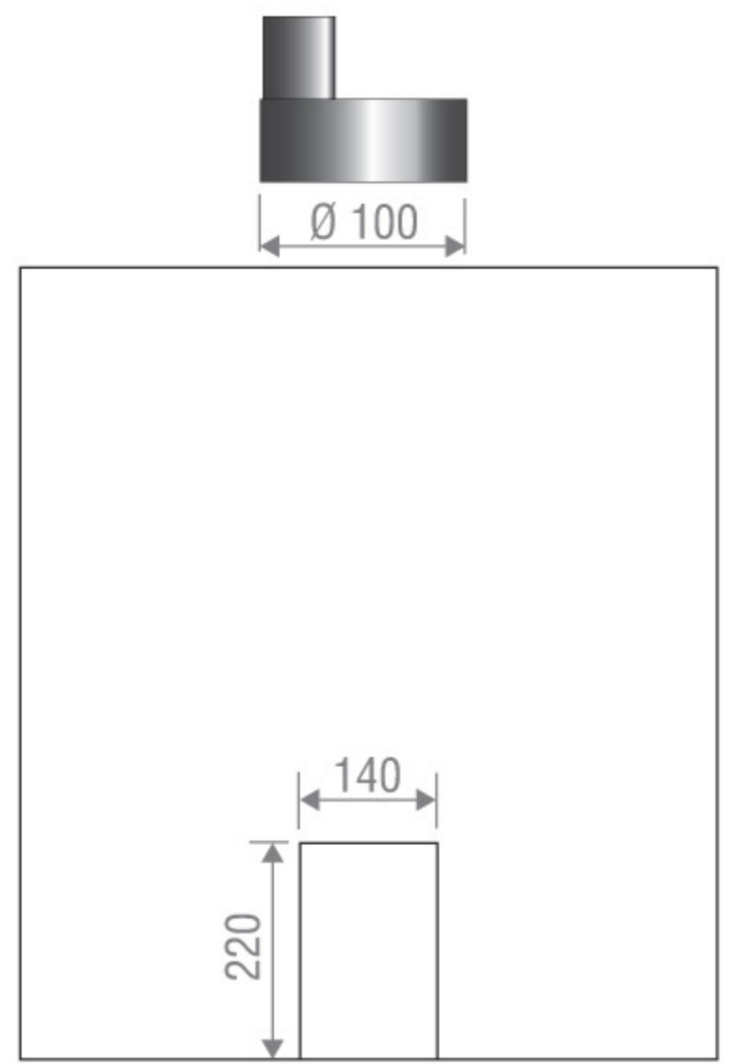
Version double combustion simple avec option adaptateur Rajout d'un bossage arrière sur convecteur Double combustion with adapter Additional rear boss on the convector
