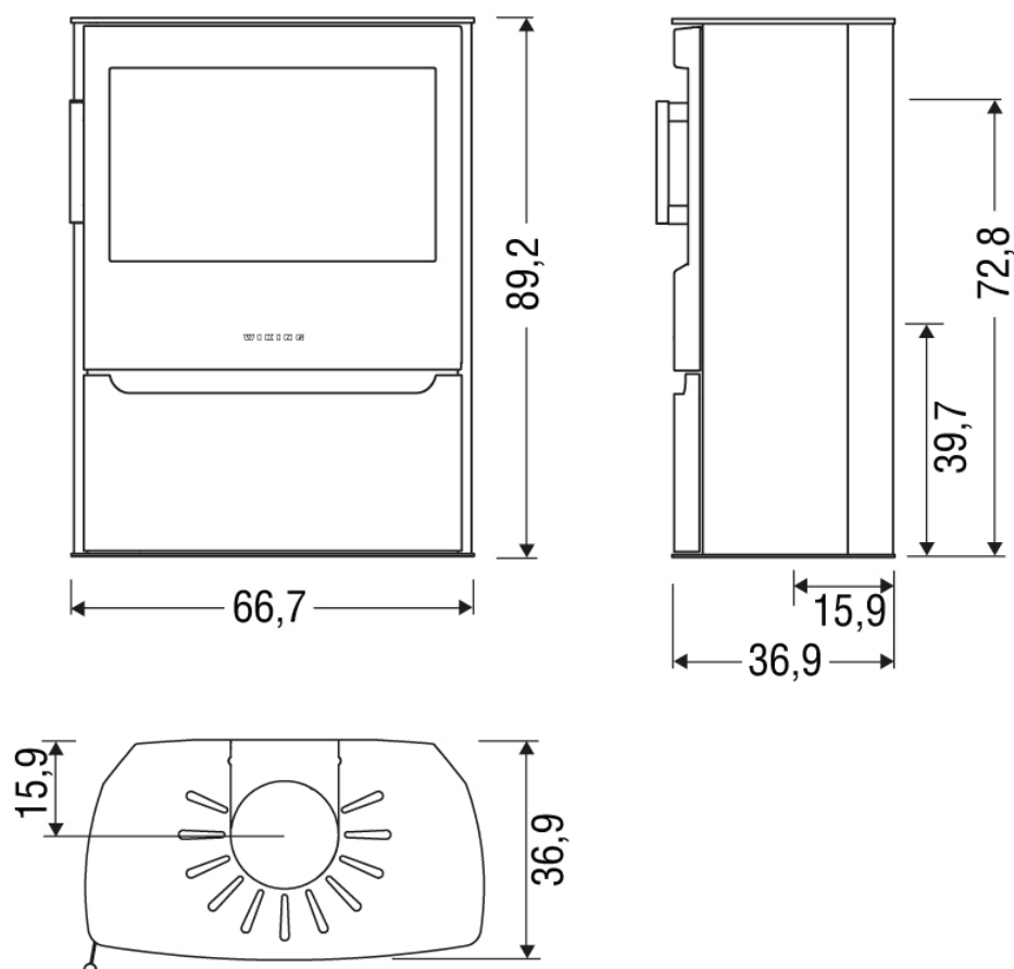
Schéma technique
