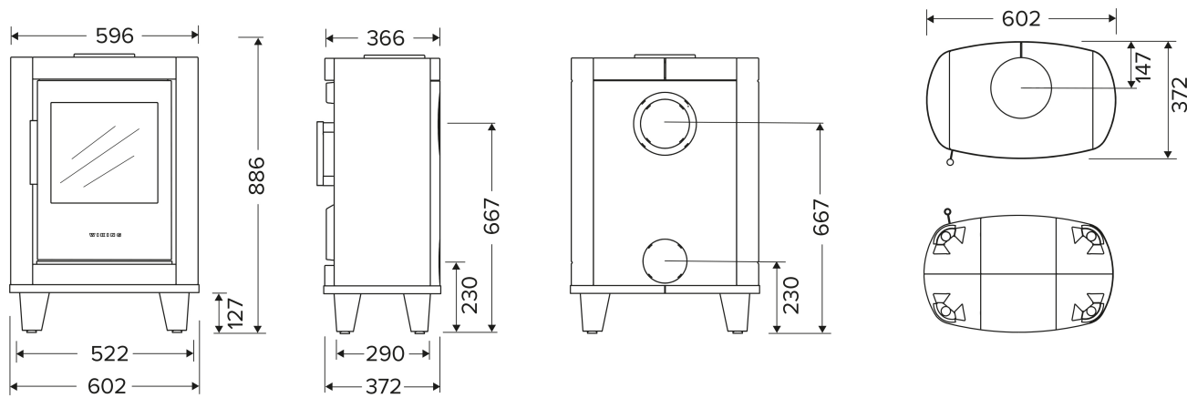
Schéma technique
